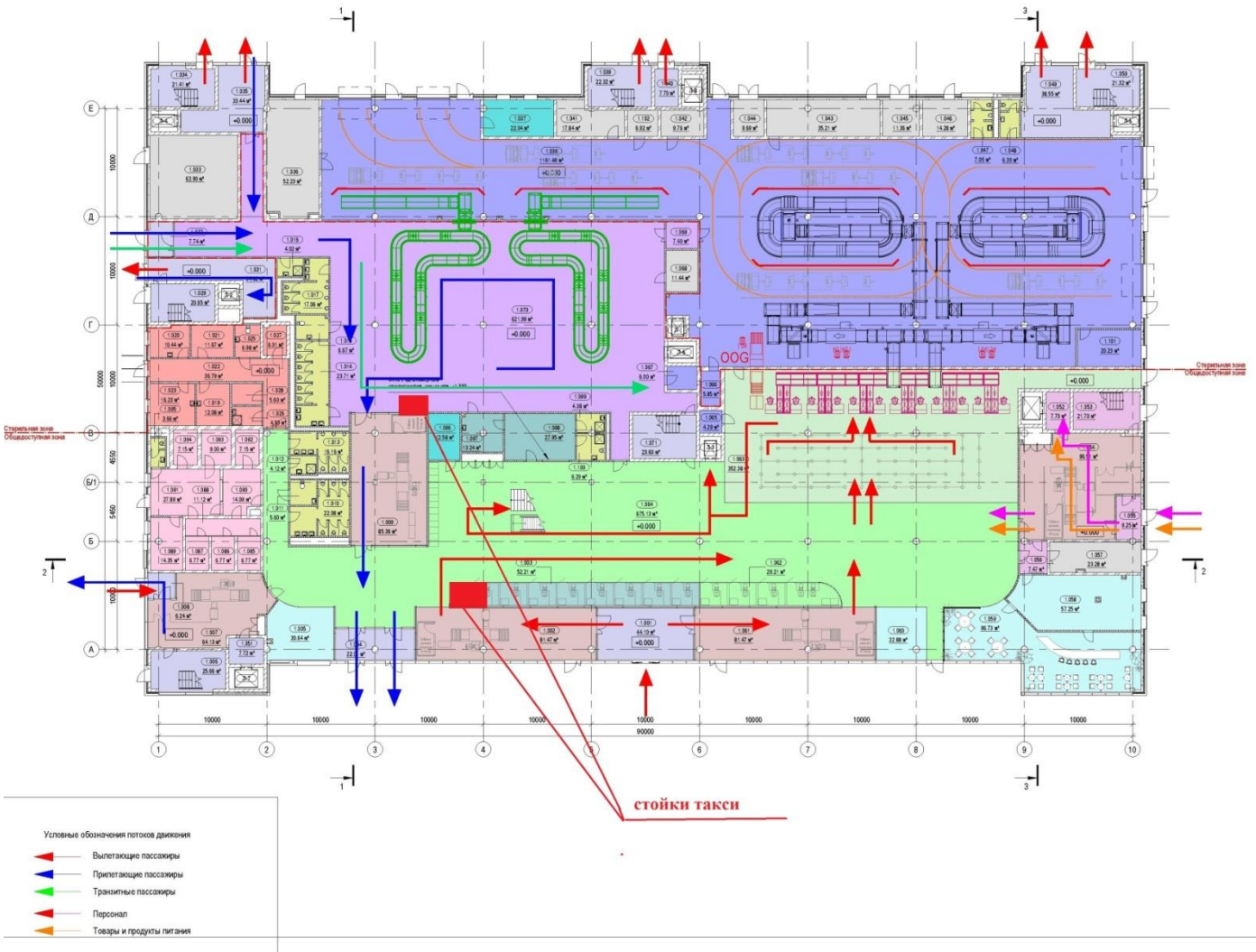
План функционального зонирования 1-го этажа (на отм. 0.000)
