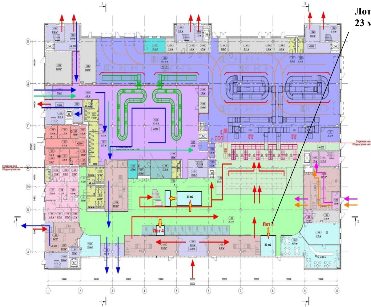
План функционального зонирования 1-го этажа (на отм. 0.000)
