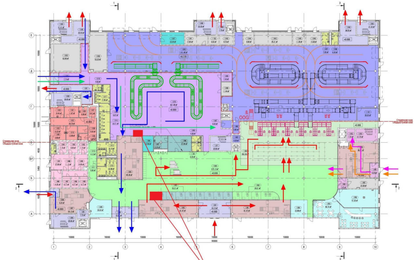
План функционального зонирования 1-го этажа (на отм. 0.000)
