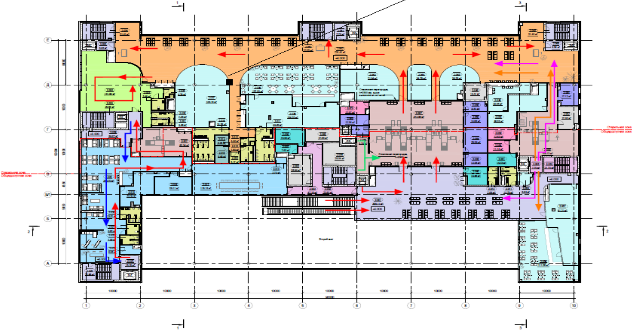
План функционального зонирования 2-го этажа (на отм. +6.000)
