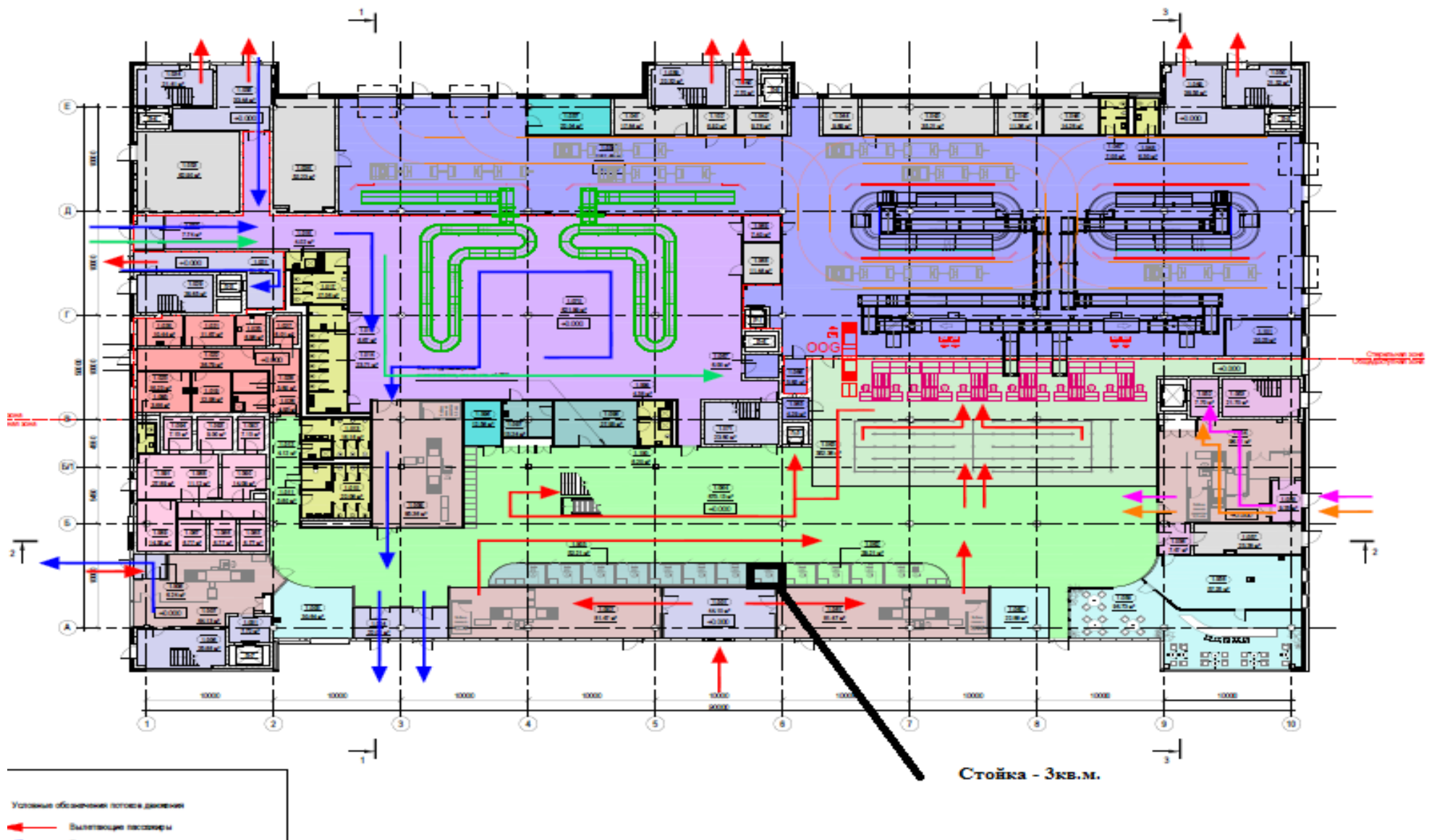
План функционального зонирования 1-го этажа (на отм. 0.000)
