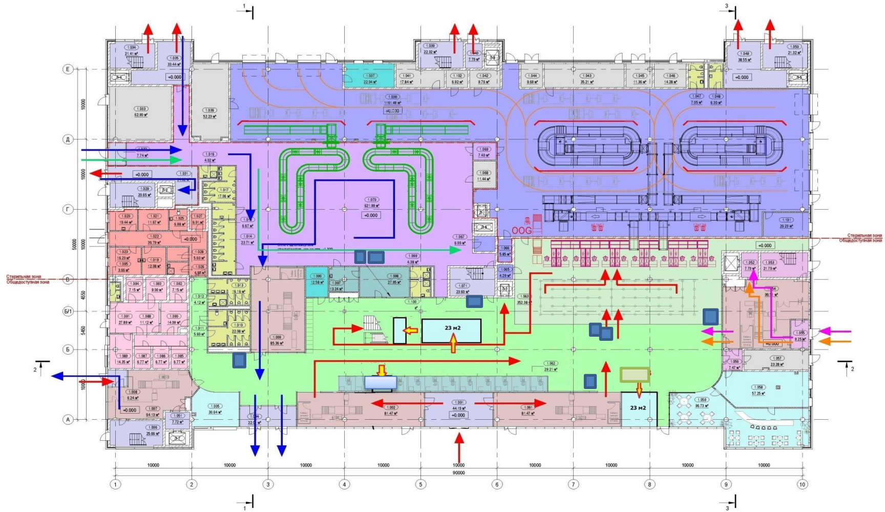
План функционального зонирования 1-го этажа (на отм. 0.000)
