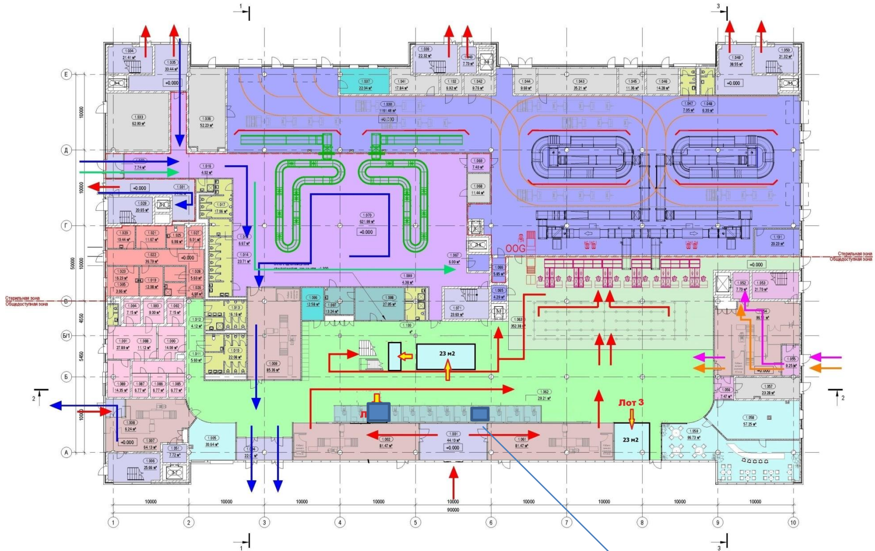
План функционального зонирования 1-го этажа (на отм. 0.000)
